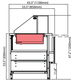
Bain Marie FRBM
